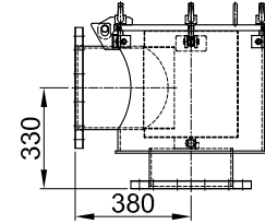
DN 250
